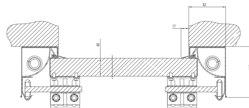
coupe horizontale de la porte sectionnelle avec ressorts de traction
